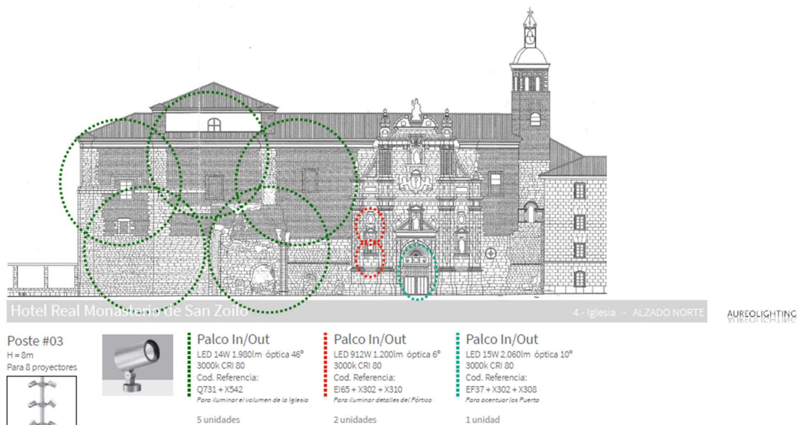
Iluminación prevista en fachada de la iglesia del monasterio de San Zoilo (Carrión de los Condes)
