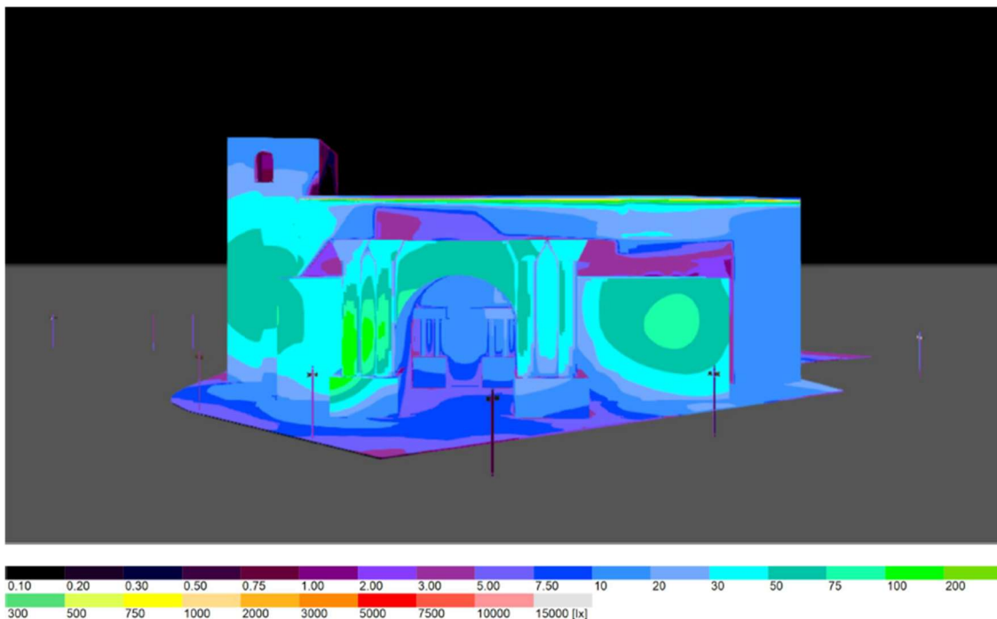
Simulación con “colores falsos” para verificación de niveles en iglesia de San Pedro (Frómista)
