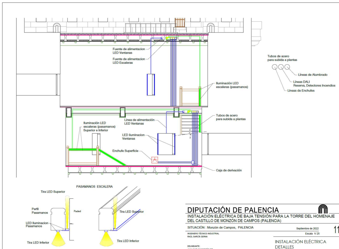
Plano de detalles del proyecto
