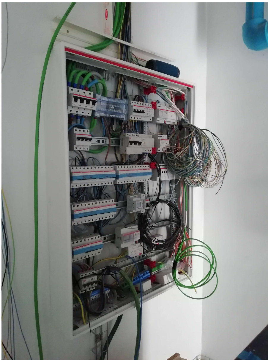
Montaje en obra de cuadro general planta baja
