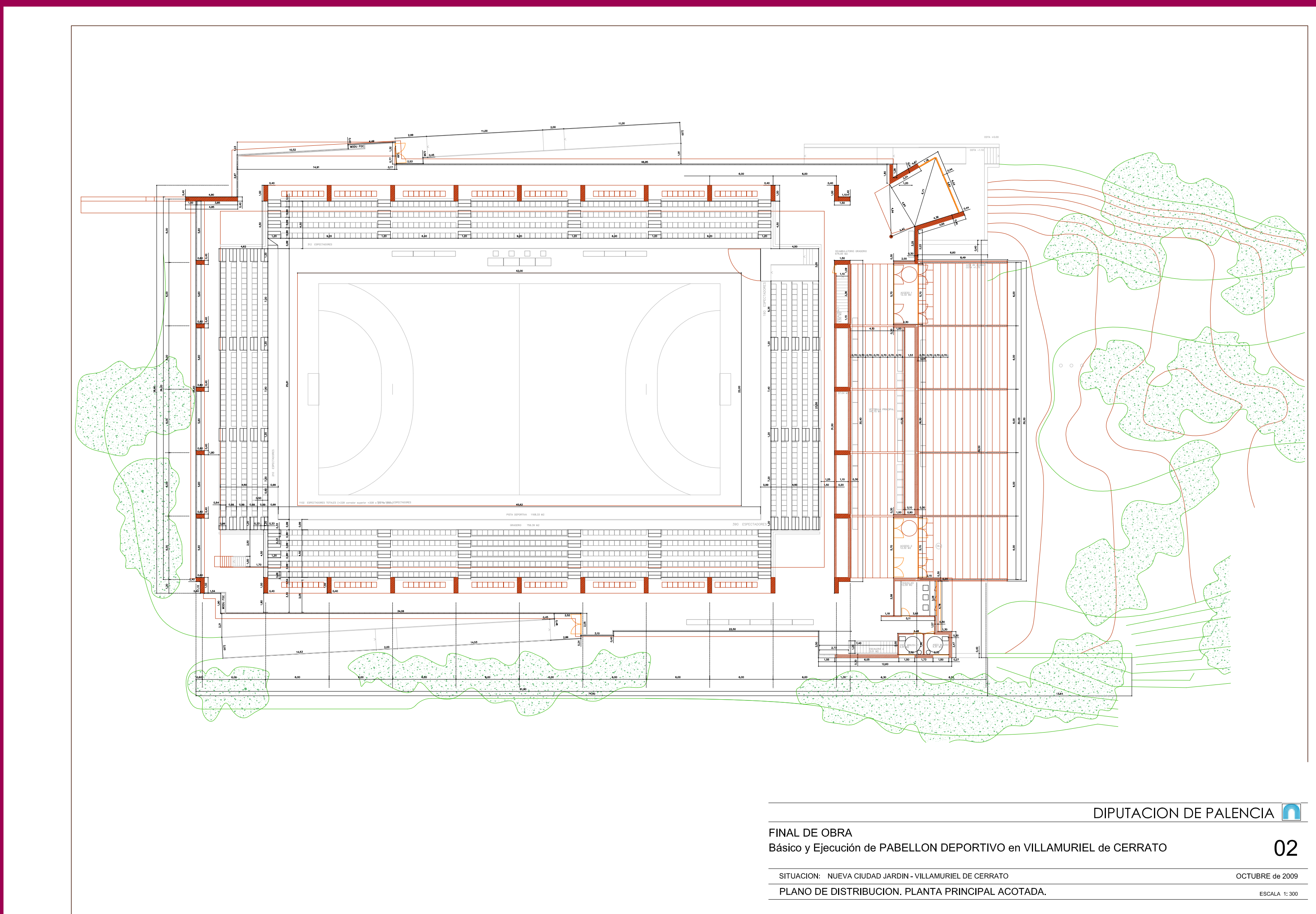
2009 Proyecto de pabellón deportivo en Villamuriel de Cerrato . - Plano de distribución Arquitectos: Gabriel Gallegos Borges Juan Carlos Sanz Blanco ADPP Archivo digital
