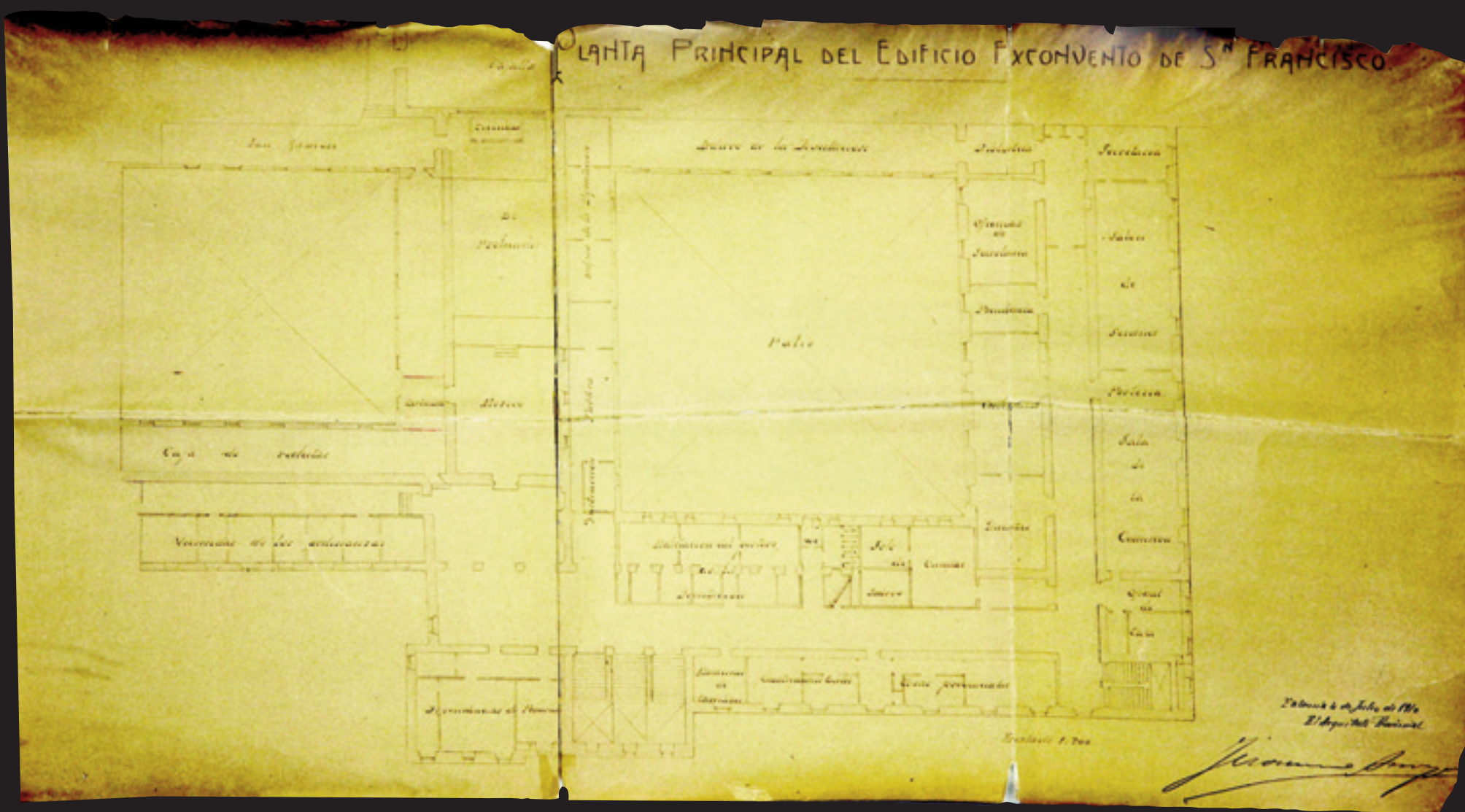
1910 Plano de Planta del Ex Convento de San Francisco, Palencia. Arquitecto Provincial: Jerónimo Arroyo. Copia en papel, 32 x 59 cm. ADPP C-1702/6
